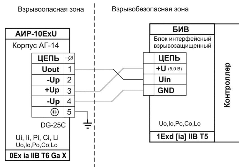
Рисунок 2.13 – Схема электрических соединений взрывозащищенных АИР-10ExP к контроллеру через БИВ в корпусе АГ-14
