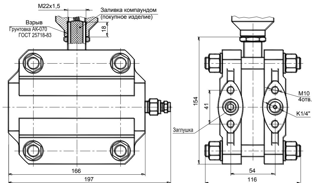
Чертеж средств взрывозащиты.
