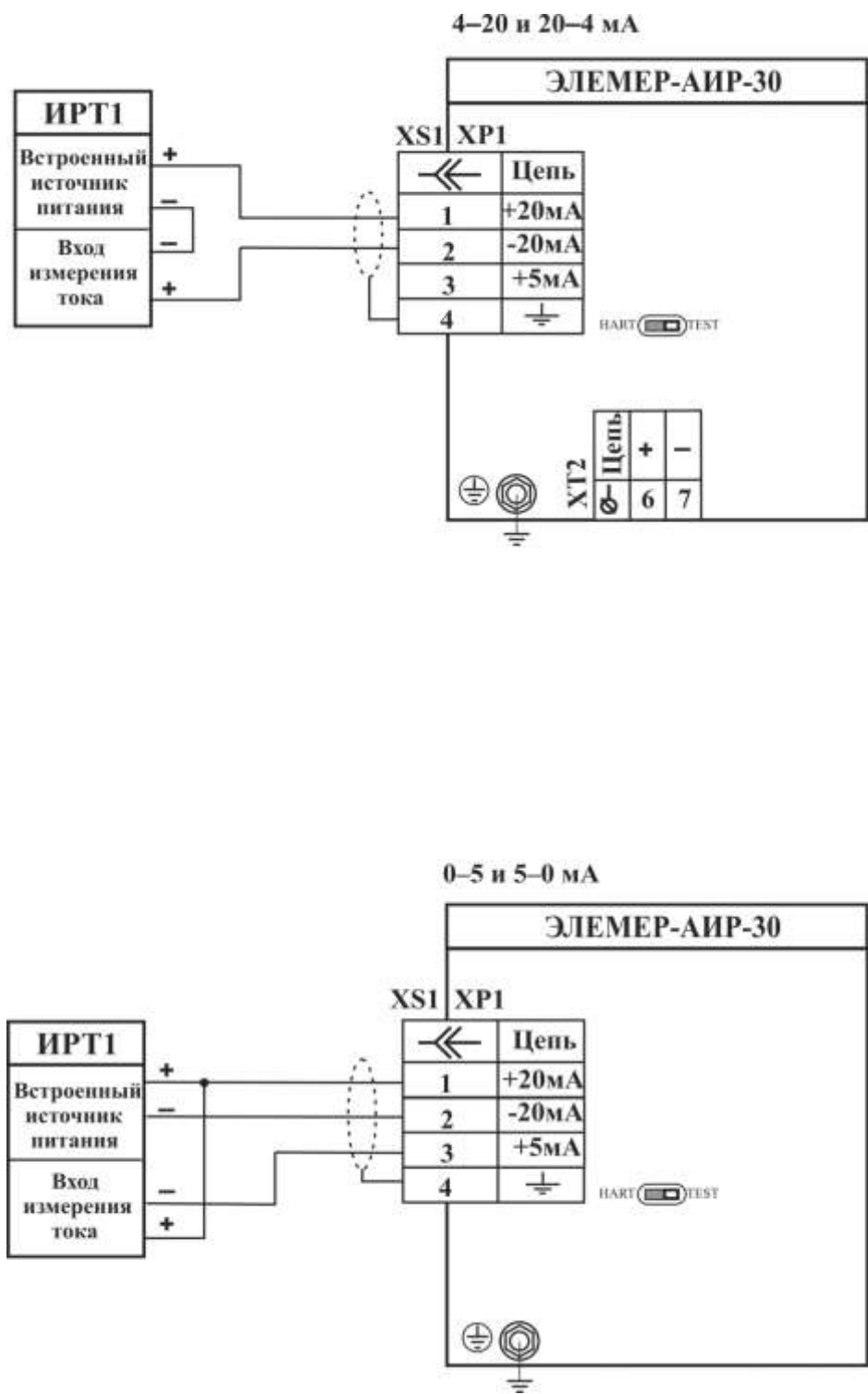
Схема электрическая подключений токовых цепей ЭЛЕМЕР-АИР-30 к различным приборам с разъёмами ШР14, ШР22 (цепи каналов сигнализации не показаны)
