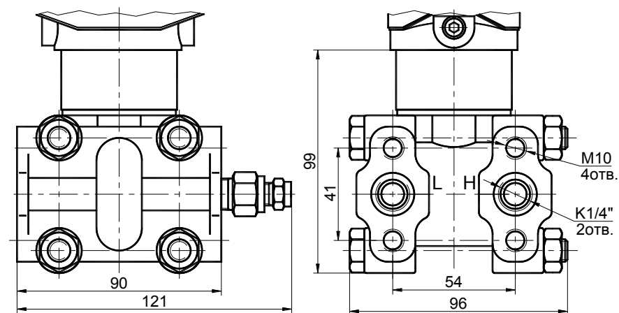
Рисунок Б.8 Габаритные и присоединительные размеры сенсоров (место Б рисунка Б.1) САПФИР-22ЕМ-ДД, САПФИР-22ЕМА-ДД
