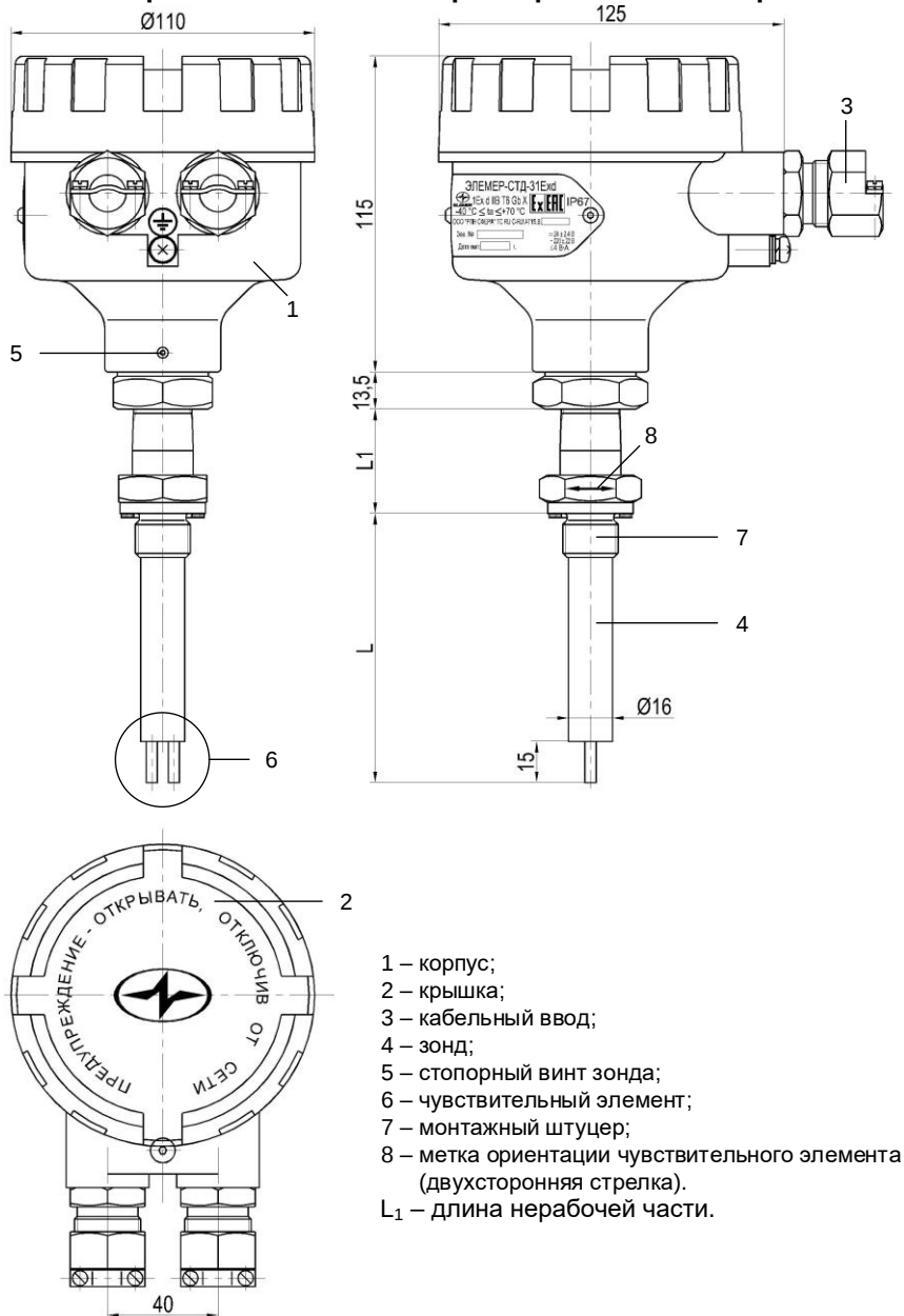
Рисунок А.1 – Габаритные и монтажные размеры сигнализаторов «ЭЛЕМЕР-СТД-31Exd»
