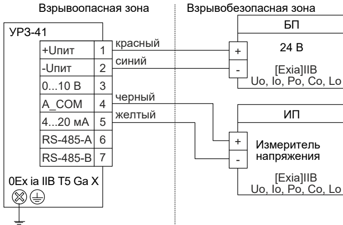
Рисунок Б.8 - Схема электрическая подключений УРЗ-41Ex (исполнение с кабельными вводами) с унифицированным выходным сигналом от 4 до 20 мА
