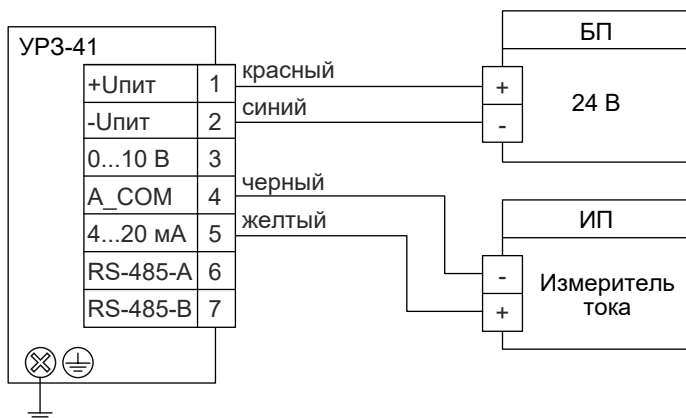
Рисунок Б.5 - Схема электрическая подключений УРЗ-41 (исполнение с кабельными вводами) с унифицированным выходным сигналом от 4 до 20 мА
