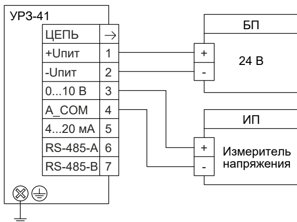
Рисунок Б.1 - Схема электрическая подключений УРЗ-41 (исполнение с разъемами) с унифицированным выходным сигналом от 0 до 10 В
