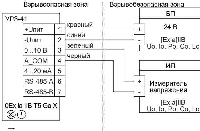
Рисунок Б.7 - Схема электрическая подключений УРЗ-41Ex (исполнение с кабельными вводами) с унифицированным выходным сигналом от 0 до 10 В
