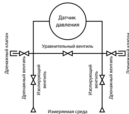
Схема подключения
