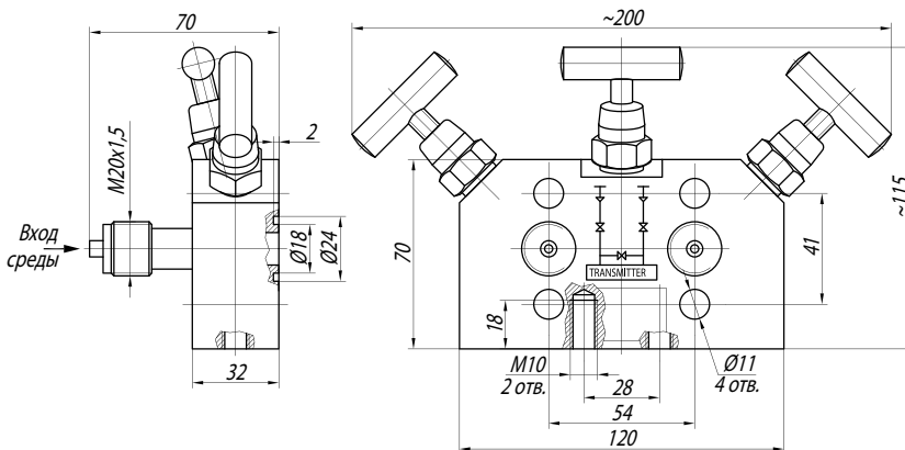
3-вентильный клапанный блок ЭЛЕМЕР-БК-С30 (без дренажа)
