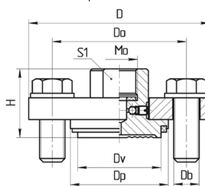
Разделитель сред типов 5320 и 5322
