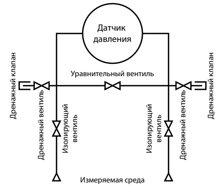
Схема подключения
