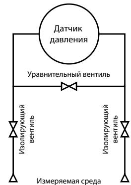
Схема подключения
